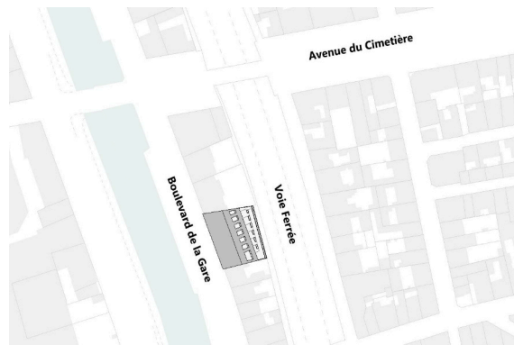
Plan masse
