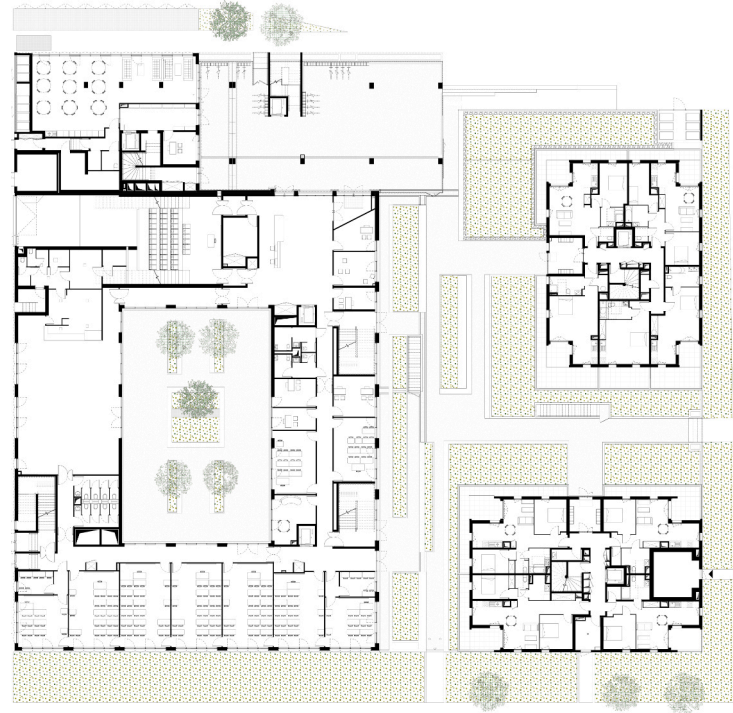
Plan RDC
